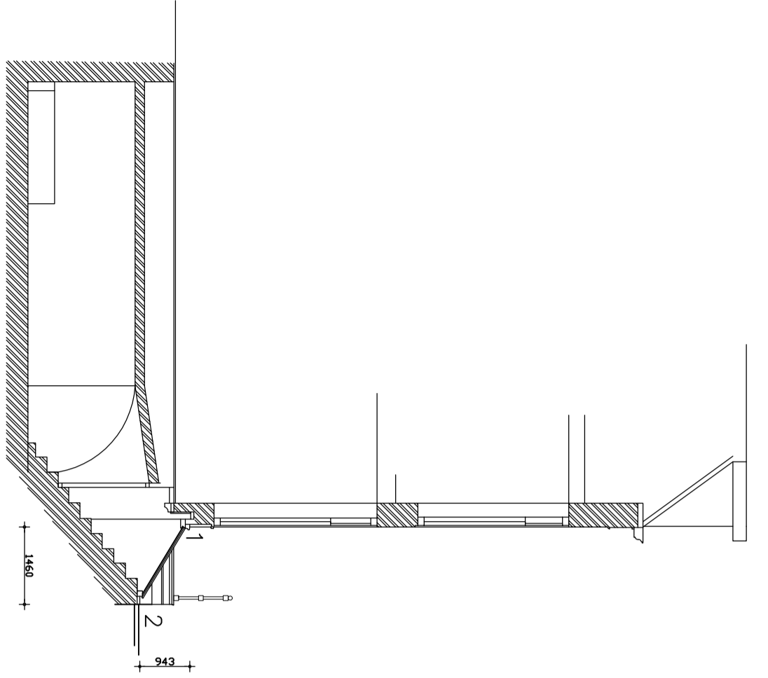
DOORSNEDE VOORGEVEL TPV Kelder
